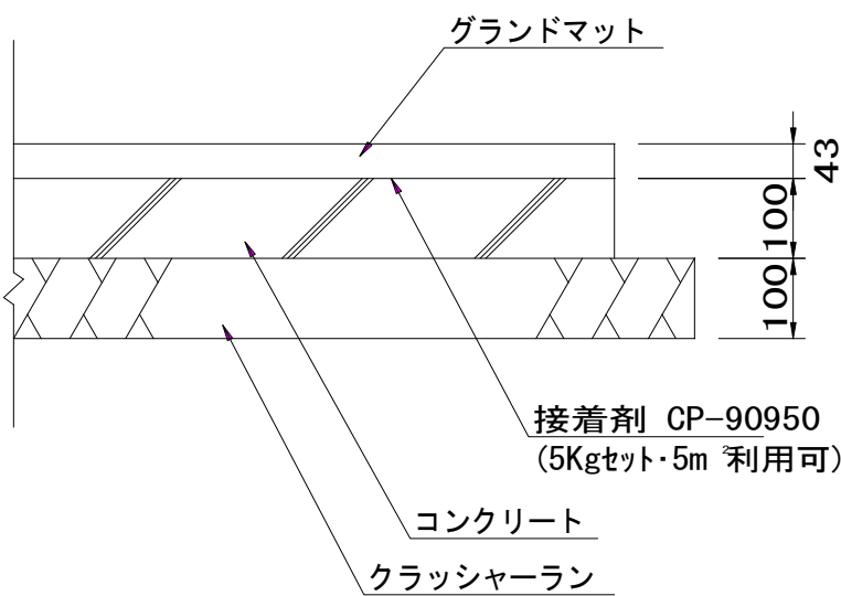
参考施工図 S = 1 / 1 0
