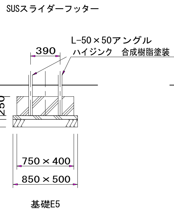
基礎詳細図 S=1/30
