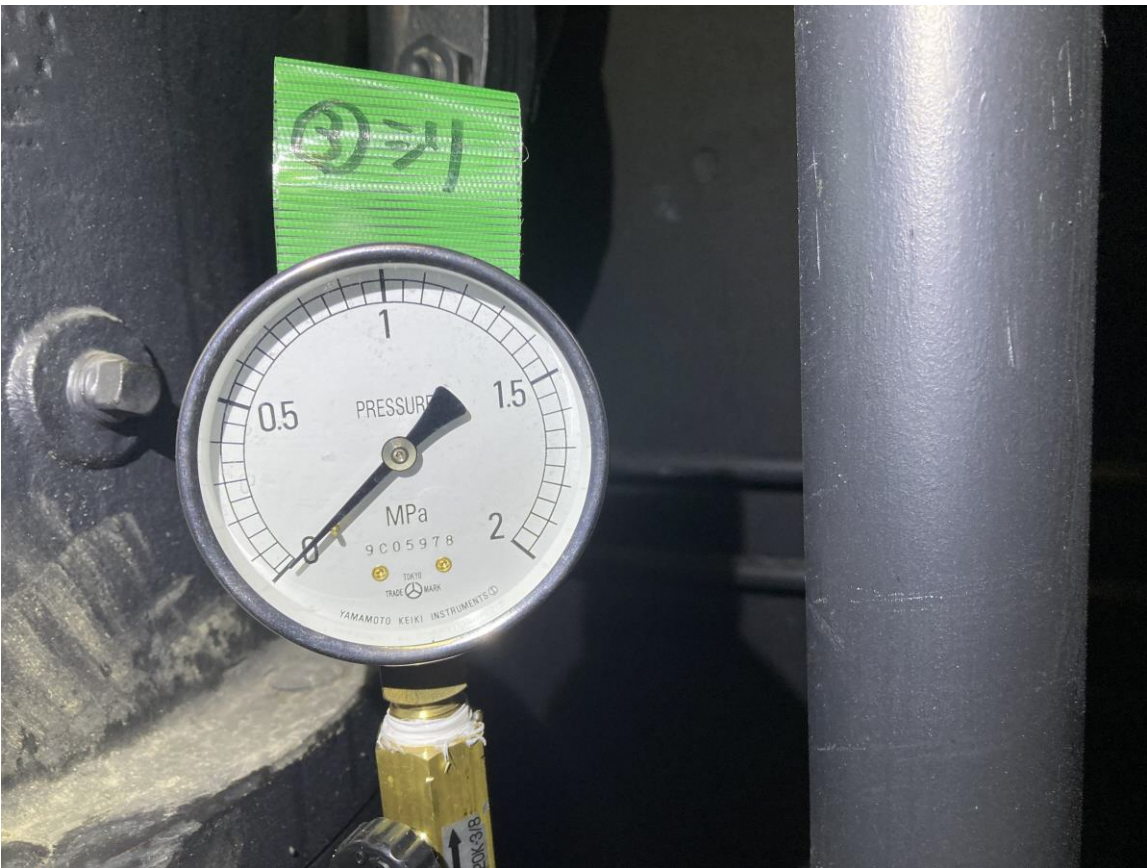
2/8から2/18まで残置した圧力計 系統3：圧力0MPa
