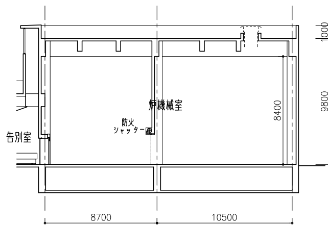
A-A'断面図 S=1/300 (A4)
