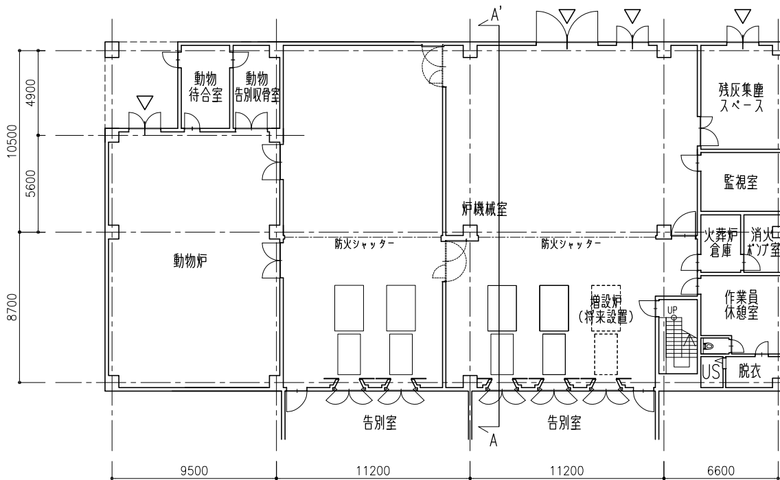
1階平面図 S=1/300 (A4)
