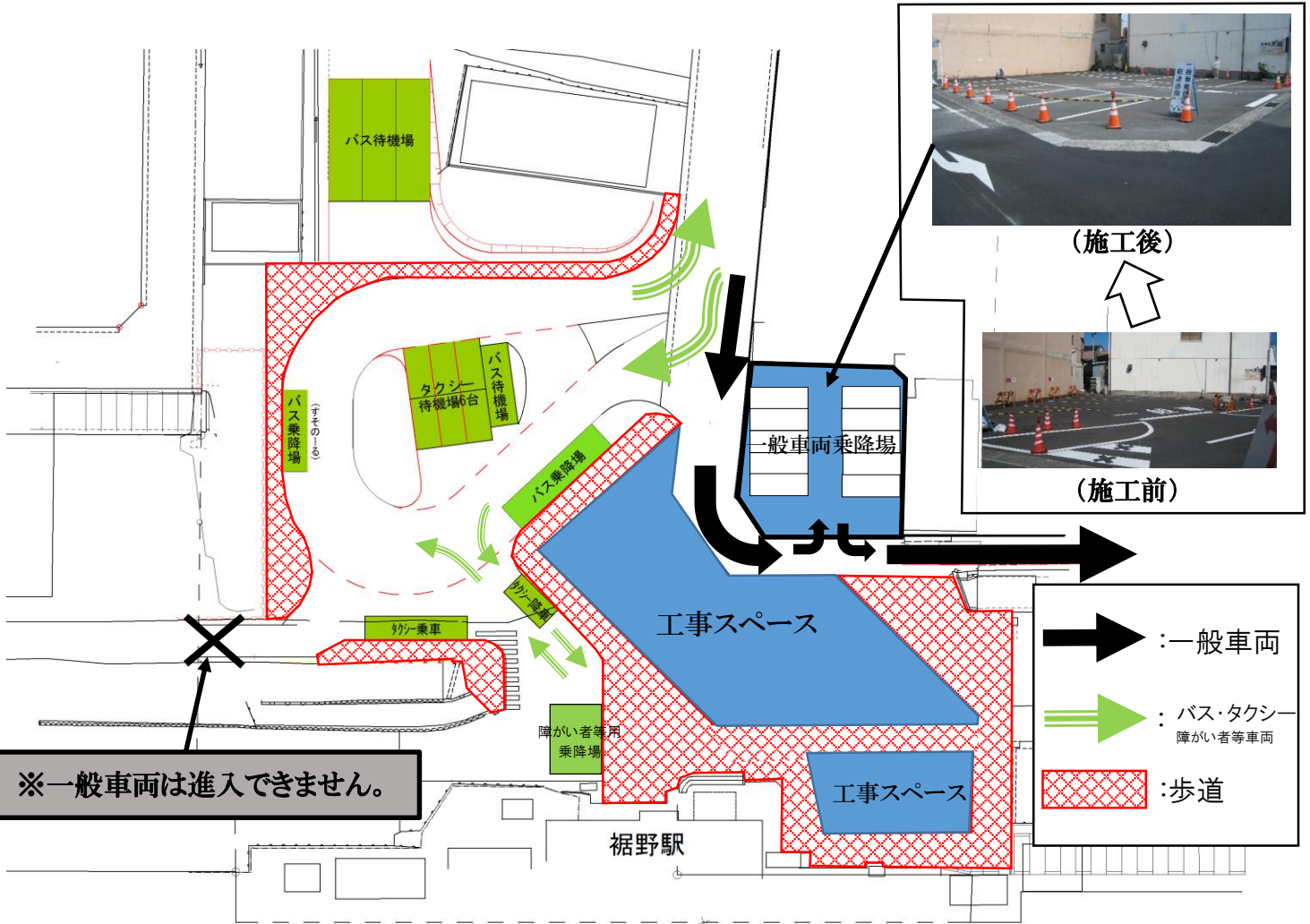
【臨時駅前広場レイアウト図】
