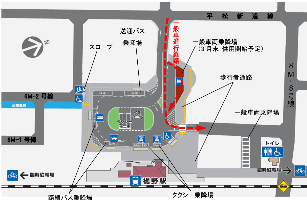
＜裾野駅西口駅前広場計画平面図＞
