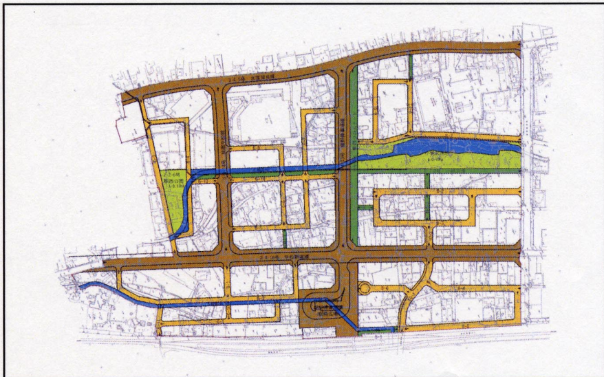
【裾野駅西土地地区画整理事業・設計図】
