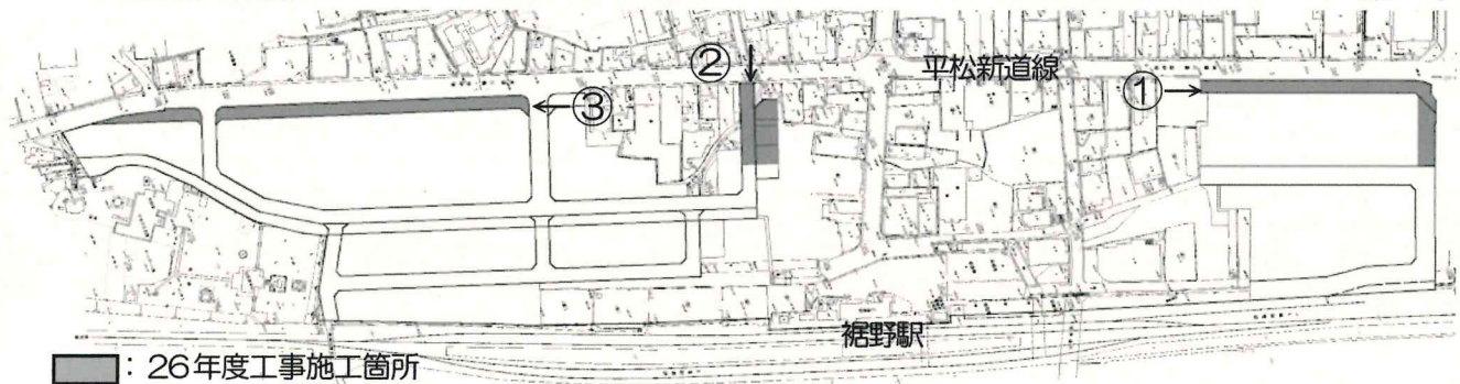
平成26年度工事箇所図
