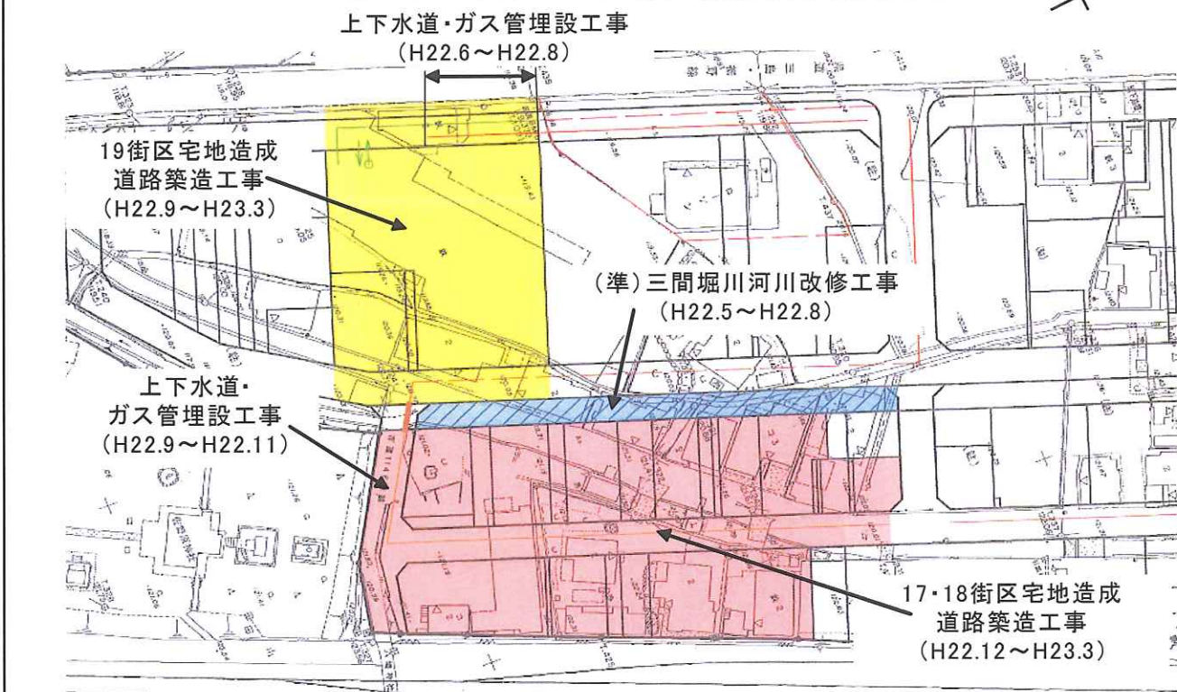
《17・18・19 街区周辺工事位置図》
