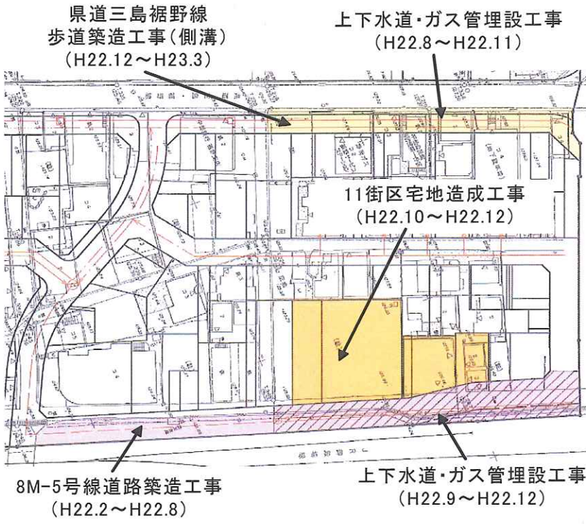
《10・11 街区周辺工事位置図》
