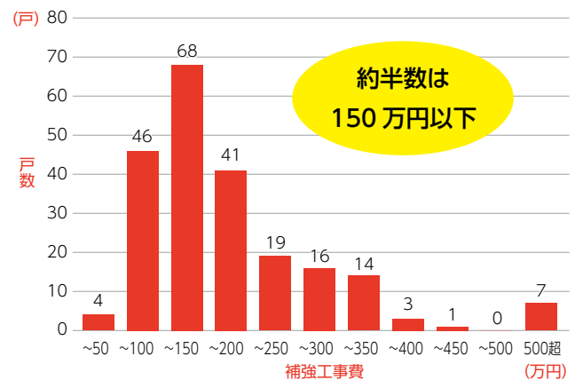
耐震補強にかかった工事費（木造住宅） （平成17～28年度）
