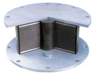
鉛プラグ入り積層ゴム
