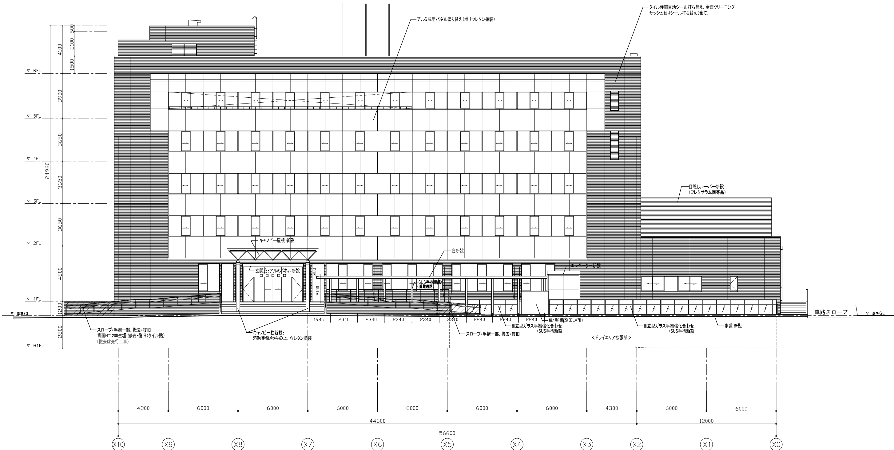
北立面図
